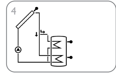
Solaranlage mit Speicherschichtbeladung (Seite 24)
