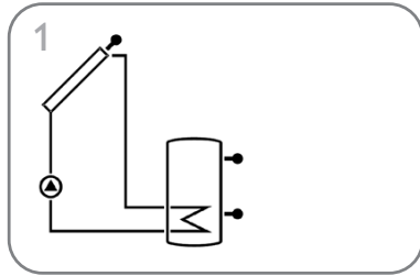
Standard-Solaranlage (Seite 10)
