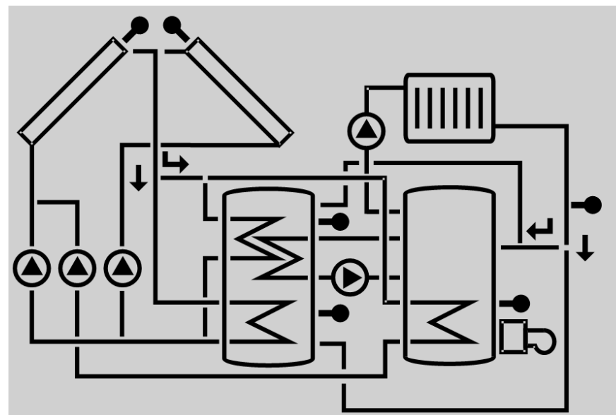
Kollektoren mit Kollektorsensor
