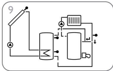
Solaranlage mit Heizkreis-Rücklaufanhebung (Seite 42)
