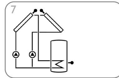
Solaranlage mit 2 Kollektoren und 1 Speicher (Seite 33)
