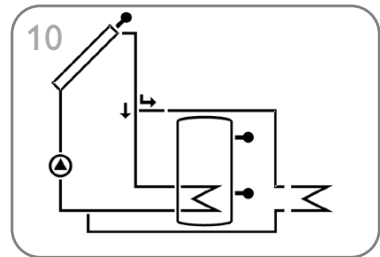
Standard-Solaranlage mit Überwärmefuhr (Seite 45)
