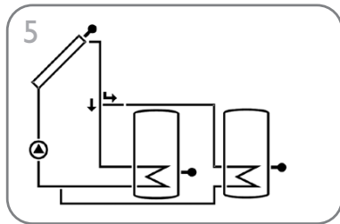
2-Speicher Solaranlage mit Ventillogik (Seite 27)
