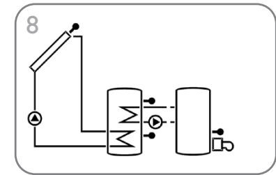
Solaranlage mit Nachheizung durch Festbrennstoffkessel (Seite 36)
