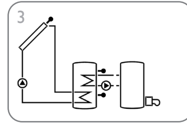
Solaranlage mit Nachheizung (Seite 19)
