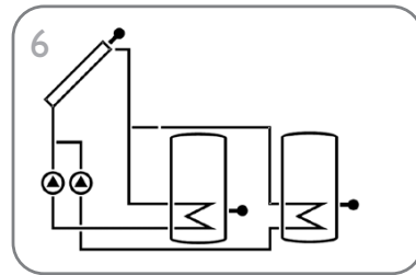
2-Speicher Solaranlage mit Pumpenlogik (Seite 30)
